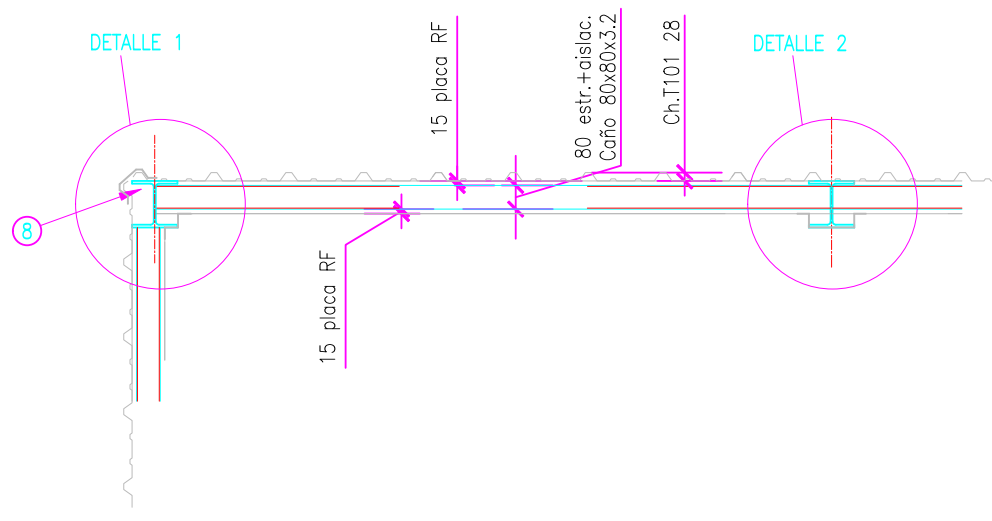
ESQUEMA DETALLE CERRAMIENTO ESCALA 1:50
