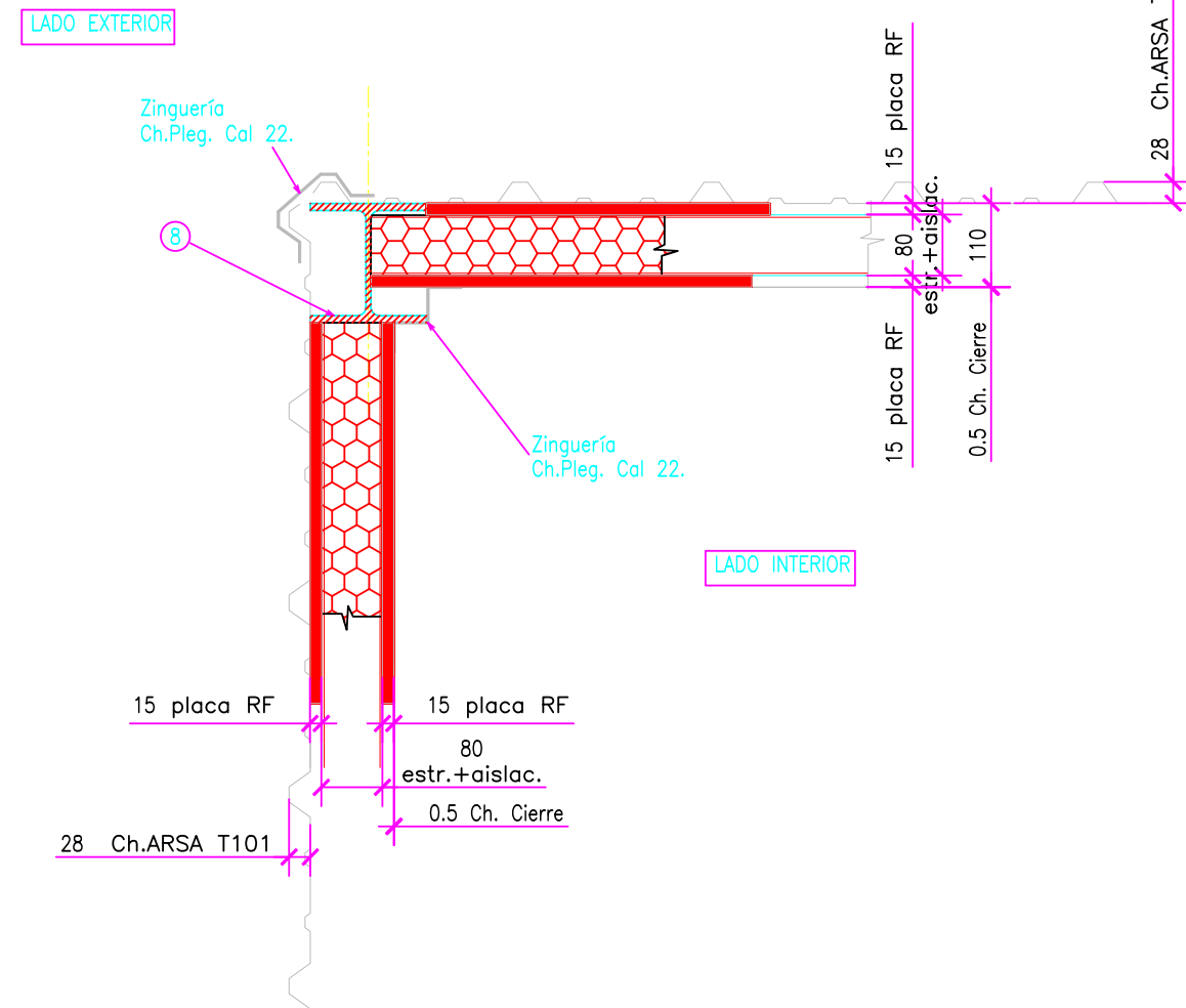
DETALLE 1 ESCALA 1:10
