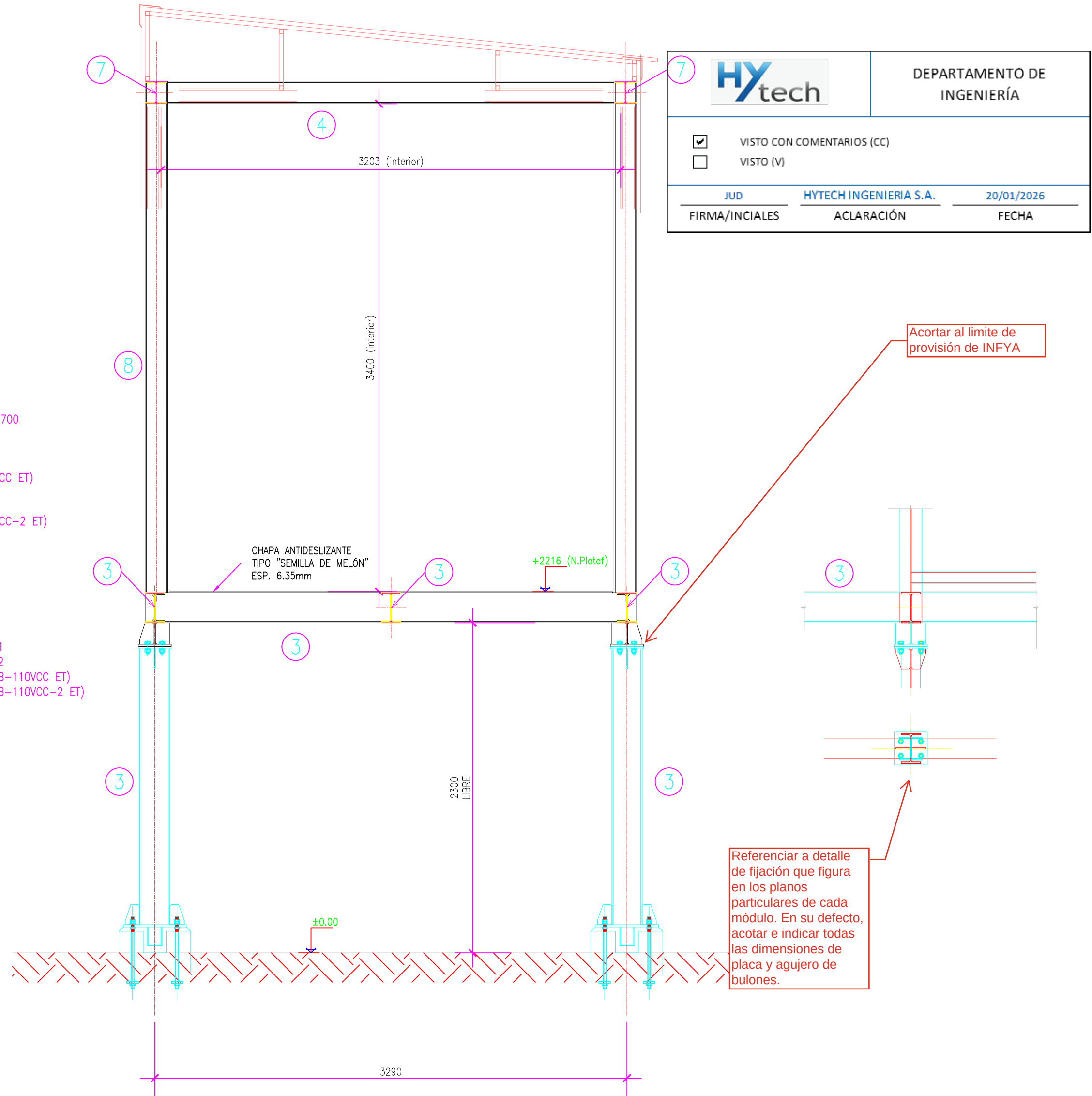
CORTE A-A ESCALA 1:25
